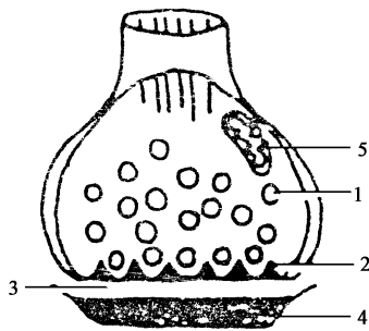
1 突触囊泡 2 突触前致密突起 3 突触间隙 4 突触后致密物质 5 线粒体 附图 Gray I型突触示意图
